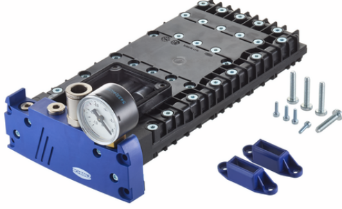
ERS FXP-SEMP-75 DECKEL
