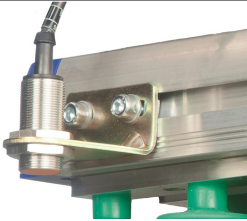
SET fuer-Sensor(FXP/FMP)
