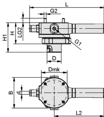
Konstruktionsdaten VEE-QCMV HV 2 07 13 SD
