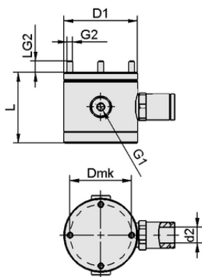
Konstruktionsdaten VEE-RU 55x55 20 FL
