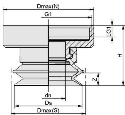
Dati di costruzione SAUG-SCG 20 SI-HD-65 602 B
