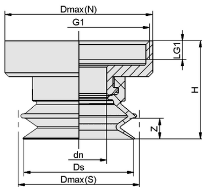
Données de construction SAUG-SCG 20 SI-HD-65 602 B
