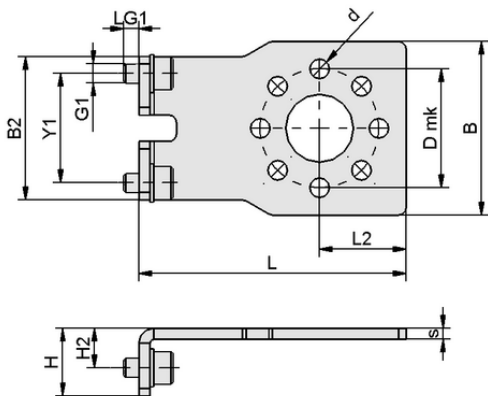
Konstruktionsdaten SET SCG-HSS MS KUKA
