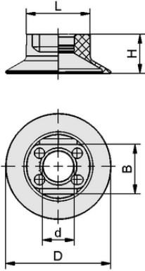
Tasarım verileri SAUG-FL SFG 59.5 36x25 POM
