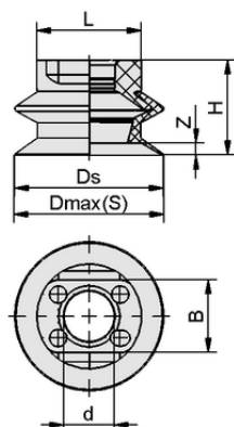
デザインデータ SAUG-SFG 40 SI-HD-65
