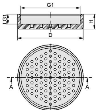
デザインデータ SAUG-FL SCGS 30 POM
