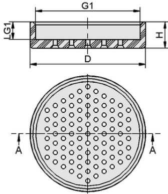
Tasarım verileri SAUG-FL SCGS 30 POM
