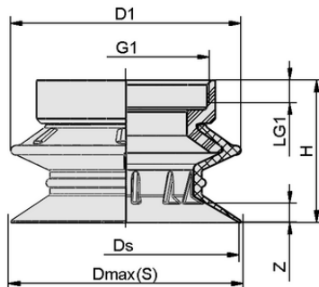
Datos de diseño SAUG-SCG 30 SI-HD-65
