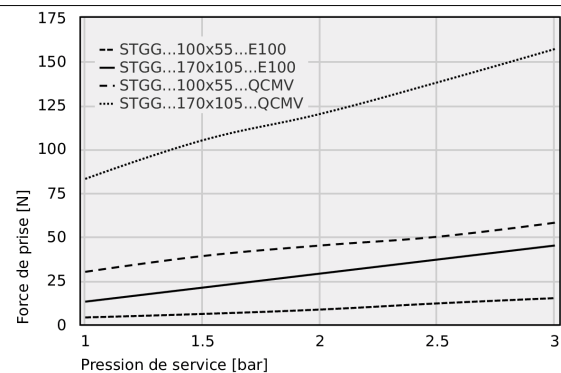
Force de pr hension
