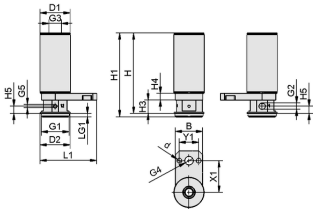
Datos de diseño SCG 1xE100 A MS SDA M37x1-AG
