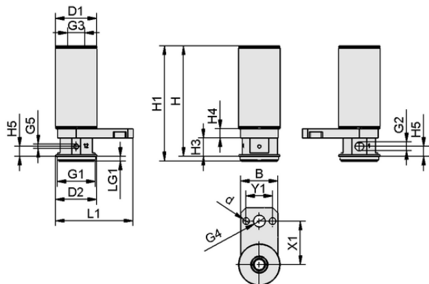
デザインデータ SCG 1xE100 A MS SDA M37x1-AG
