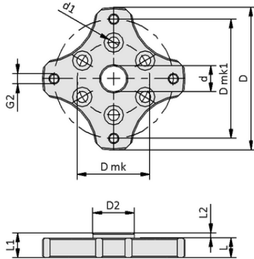
Tasarım verileri FLAN-PL 55x7.5-EL1
