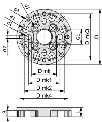
Données de construction FLAN-PL 55x9.5-JP1
