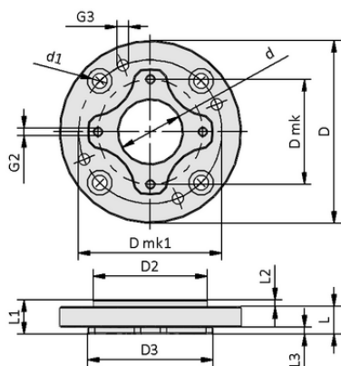
Konstruktionsdaten FLAN-PL 80x12-ST1
