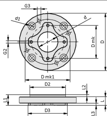
デザインデータ FLAN-PL 80x12-ST1
