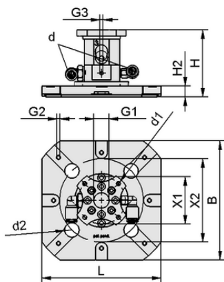
Datos de diseño SWGm-5S 115x115x65 1xE100 A PEEK
