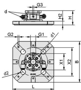
Données de construction SWGm-5A 115x115x40 1xE100 A PEEK
