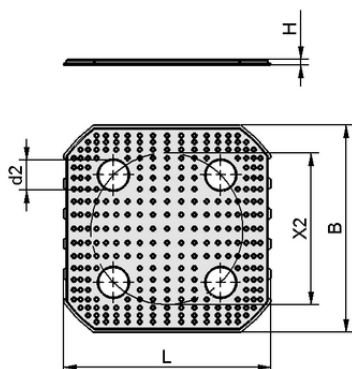
Konstruktionsdaten SAUG-FL SWGm-6 141x141 PEEK
