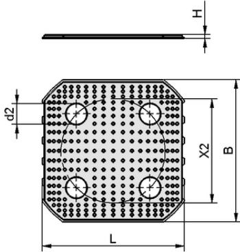
Tasarım verileri SAUG-FL SWGm-6 141x141 PEEK
