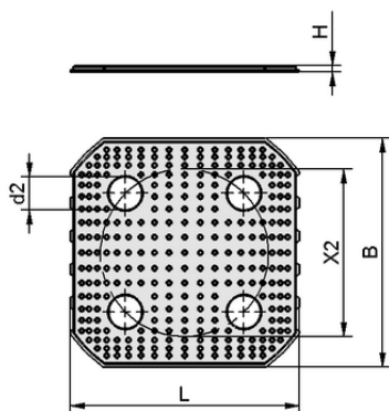
デザインデータ SAUG-FL SWGm-5 110x110 PEEK
