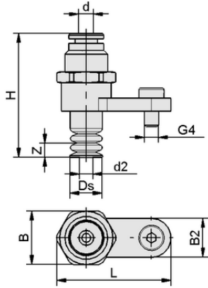
Tasarım verileri SD-MOD 4 32x15x35 FG 9 SWGm
