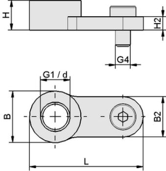
Tasarım verileri HTR M12x1-IG SWGm
