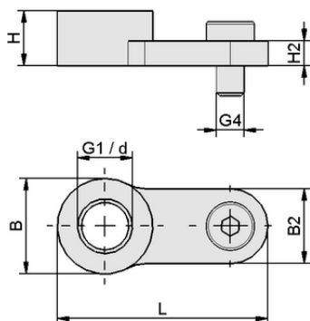
Datos de diseño HTR M12x1-IG SWGm
