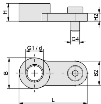
Données de construction HTR M8x1-IG SWGm
