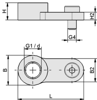
Datos de diseño HTR M8x1-IG SWGm
