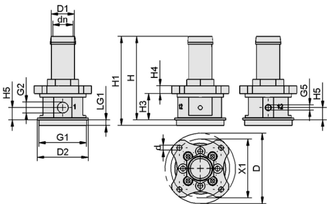
Datos de diseño SCG 1xE100 A MA AR M37x1-AG
