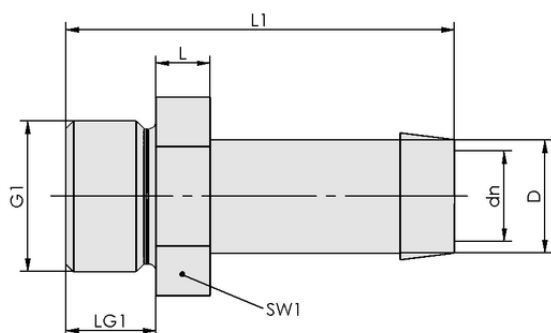
デザインデータ ABL-FUEHR 18x46 SWGm/SCG
