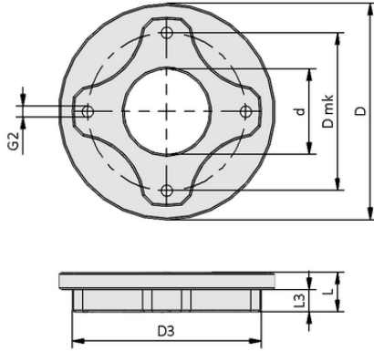
Tasarım verileri FLAN-PL 63x11.5-UNI
