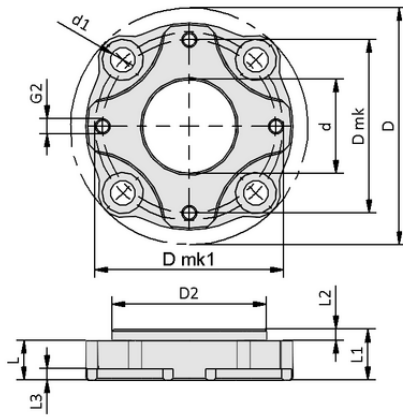
Tasarım verileri FLAN-PL 63x10.5-AD1
