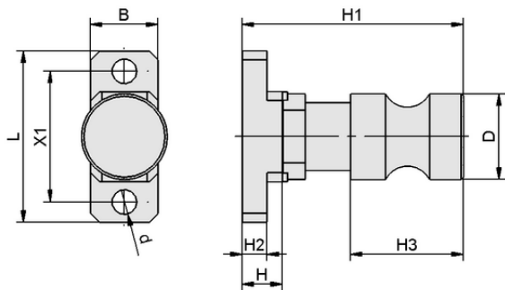
Design data HTS-A2 SNG AP/AE OP
