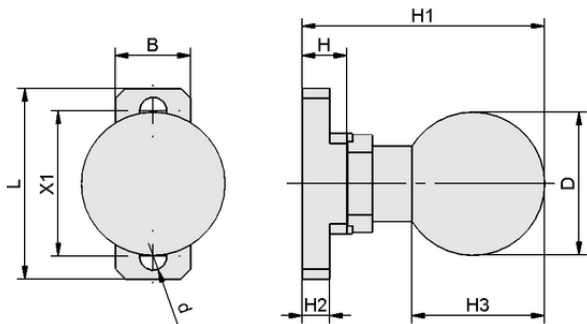
Design data HTS-A3 SNG AP/AE OP
