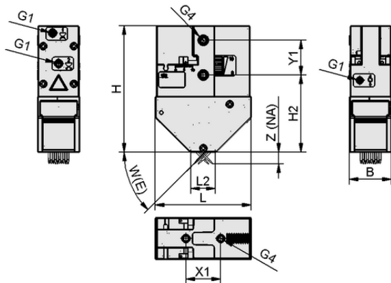
Dati di costruzione SNG-AP 10 1.2 V 10
