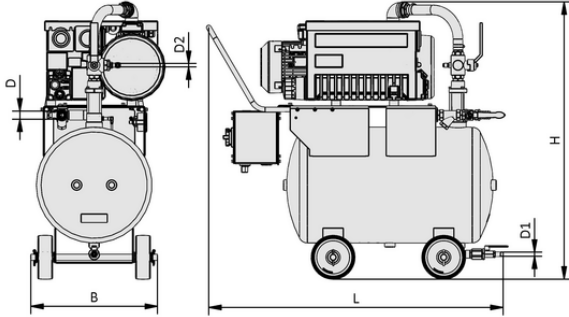
Tasarım verileri VAGG 63 AC3 80 MD
