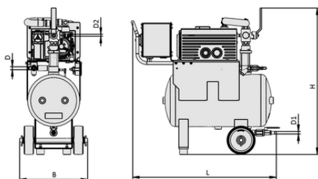
Dati di costruzione VAGG 10 AC3 30 MD
