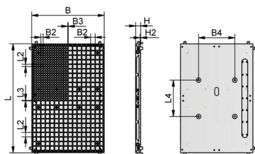
Konstruktionsdaten MPL 300x200x28 12,5x12,5 3x3
