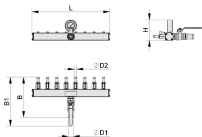
Конструктивные данные VTR-ZF 8x 1TN MAN/KVZ
