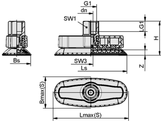
Tasarım verileri SAOXM 60x20 ED-85 G1/4-IG
