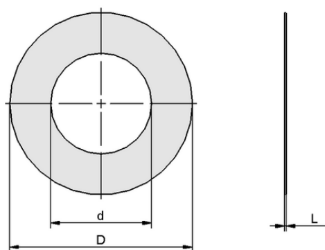
Données de construction DR-SPL-HT 35 ST
