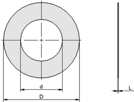
Tasarım verileri DR-SPL-HT 35 ST
