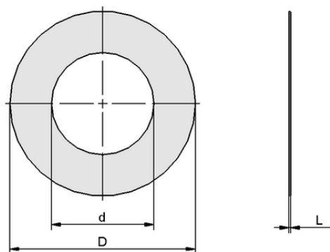
Datos de diseño DR-SPL-HT 90 ST
