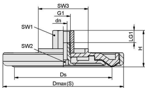
Dati di costruzione SPL-HT 90 ST G1/4-IG
