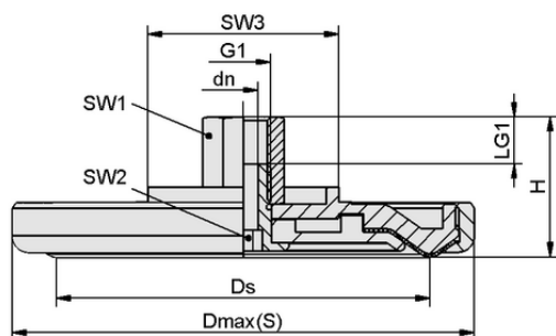
Datos de diseño SPL-HT 60 ST G1/4-IG
