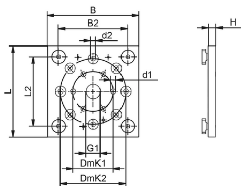
Конструктивные данные SET FXC-FMC
