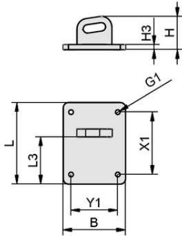
Tasarım verileri MOD-FLAN 157x120 SBX-C
