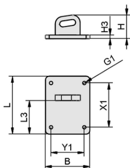
Datos de diseño MOD-FLAN 157x120 SBX-C
