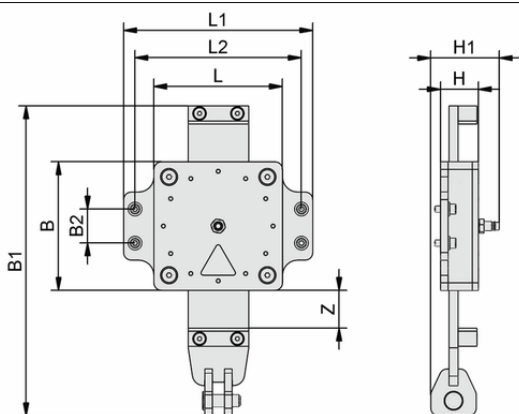
Datos de diseño FST-C 100-HD1
